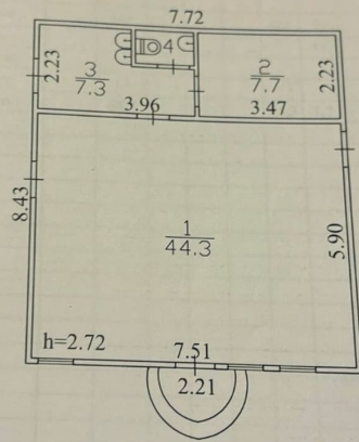
План строения
