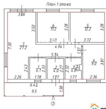
План этажа (части этажа), План объекта недвижимости (части объекта недвижимости)
